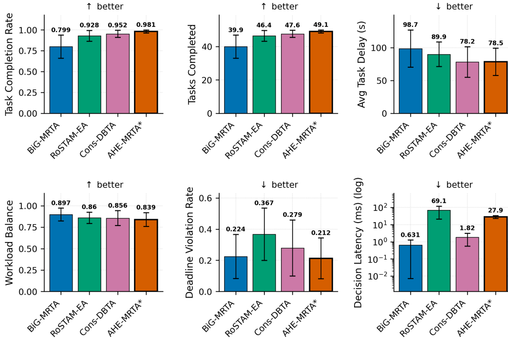
Fig. 8. 10-robot ölçeğinde çok-metrikli karşılaştırma (60 deney: 4 yöntem \times 3 senaryo \times 5 tohum; üç senaryo havuzlandığı için her çubuk n=15 ; ortalama \pm standart sapma; karar gecikmesi log ölçek). Senaryolar üzerinden havuzlandığında AHE-MRTA tamamlamada öndedir (0.799–0.952’ye karşı 0.981) ve deadline ihlalinde en düşüktür (0.224–0.367’ye karşı 0.212); ortalama karar gecikmesi ise commit-once temel yöntemlerin 0.6–1.8 ms’sine ve RoSTAM-EA’nın 69.1 ms’sine karşı 27.9 ms’dir. Havuzlama, deadline marjının nereden geldiğini gizler: marj deadline_pressure ’da yoğunlaşır (0.296–0.504’e karşı DVR 0.220) ve metin bunu senaryo bazında raporlar. Senaryo başına n=5 ’lik çapraz-yöntem hücreleri betimleyicidir, düzeltilmiş bir sıralama kurmaz.
