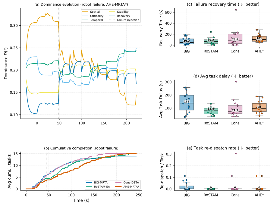
Fig. 11. robot_failure altında yorumlanabilir uyum (3r/15g). Zaman, her koşunun ilk görev etkinleşmesinden ölçülür; böylece (a) ve (b)'deki enjeksiyon işaretleri senaryonun 45 \pm 5 s'lik ofsetine oturur. (a) Temsili bir AHE-MRTA koşusunun hormon baskınlığı; arıza öncesi evreye uzamsal hormon liderlik eder ( D \approx 0.31 ) ve enjeksiyonda (noktalı çizgi, t \approx 49 s) çöker, buna karşılık toparlanma ve kararlılık hormonları yükselir ( 0.12 \rightarrow 0.20 ve 0.15 \rightarrow 0.20 ). Sonrasında hiçbir hormon arıza öncesi farkı geri kazanmaz: koşunun kalanına kritiklik ve zamansal kanallar liderlik eder, gönderilen paradigma zamansal, uzamsal ve toparlanma geçişleri arasında dönüşümlü çalışır. (b) Kümülatif görev tamamlama (tohum-ortalama; noktalı çizgi: medyan enjeksiyon t \approx 44 s): AHE-MRTA arızadan sonra tamamlamaya devam eder ve tam görev kümesine ulaşır; ancak üç reaktif yöntem içinde buna en son ulaşan odur. (c–e) Toparlanma süresi, ortalama görev gecikmesi ve görev yeniden-gönderim oranı kutu grafikleri (kutu: IQR; çizgi: medyan; bıyıklar: 1.5 \times \text{IQR} ; noktalar: tekil koşular, yöntem başına n=15 ): AHE'nin reaktifliği en yüksek toparlanma-süresi medyanı olarak görünür (49–77 s'ye karşı 101 s); gecikme medyanı (98 s) uzlaşma temel yöntemleri (72–84 s) ile görev-terk eden BiG-MRTA (138 s) arasındadır ve yeniden-gönderim medyanı dört yöntemde de sıfırdır.
