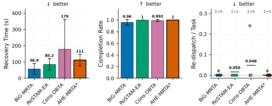
Fig. 10. Birincil 5-robot / 25-görev ölçeğinde robot_failure altında arıza-toparlanma davranışı ( n=5 tohum): toparlanma süresi ile tamamlama oranı (ortalama \pm std çubukları; bıyıklar sıfırda kırpılmıştır) ve yeniden-gönderim oranı — 20 koşunun 17'si tam sıfır olduğundan ve ortalama çubuğunu tek bir tohum taşıyacağından bu panel tohum-başına noktalar, ortalama çizgisi ve yöntem başına toplam olay sayısı ( \Sigma ) ile gösterilmiştir (yürütme kesintileri tüm yöntemlerde sıfır olduğundan gösterilmedi). Toparlanma süreleri yöntemler arasında istatistiksel olarak ayırt edilemez ( p>0.3 ); yeniden-gönderim yalnız iki temelde görülür (RoSTAM-EA: iki tohumda birer, Cons-DBTA: tek tohumda altı) ve AHE-MRTA, karşılaştırılabilir toparlanma süresini bir ekosistem güncelleme çevrimi içinde ( \leq 2 s) yetim-kurtarma paradigmasına geçerek reaktif yöntemlerin en yüksek tamamlama oranına çevirir.
