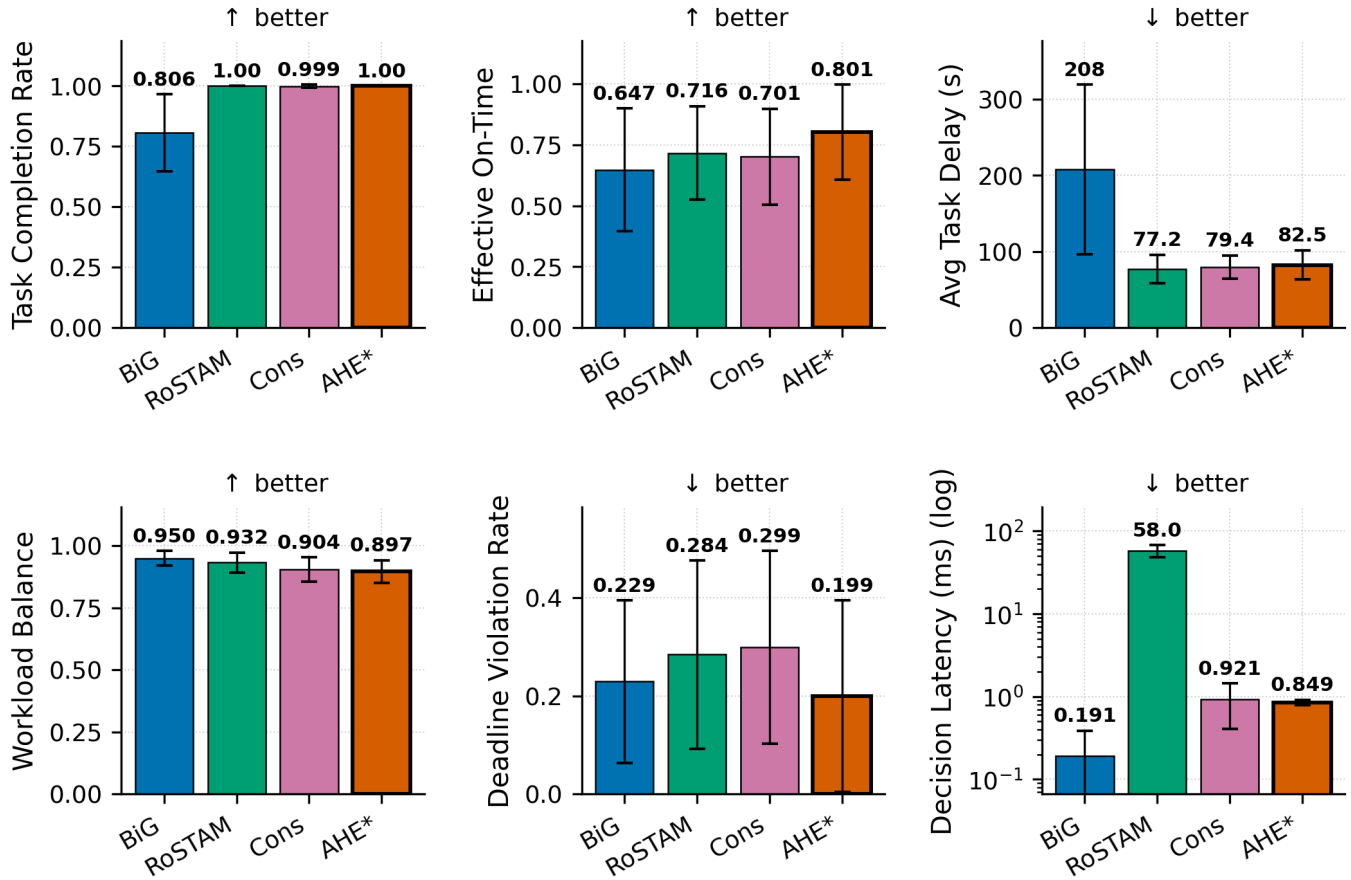
Şekil 9. Birincil 5-robot/25-görev ölçeğinde çok ölçütlü karşılaştırma. robot_failure ve mixed_stress senaryoları gösterim amacıyla birleştirilmiştir. Her yöntem-senaryo hücrelerinde n=20 tohum bulunur ve çubuklar ortalama \pm standart sapmayı gösterir. Ölçütler tamamlama oranı, zamanında etkin tamamlama CR \times (1 - DVR) , ortalama gecikme, Jain iş yükü dengesi, son teslim ihlal oranı ve logaritmik ölçekle karar gecikmesidir. AHE-MRTA CR = 1.000 ve 0.801 zamanında etkin tamamlama elde eder. Diğer yöntemlerde ikinci ölçüt 0.647-0.716 aralığındadır. BiG-MRTA'nın düşük DVR değeri en düşük tamamlama oranıyla birlikte değerlendirilmelidir. AHE-MRTA'nın reaktif yeniden tahsisi daha yüksek gecikme ve rota maliyetiyle ilişkilidir. Düzeltilmiş testler her senaryoda ayrı yürütülmüş ve metinde raporlanmıştır.
