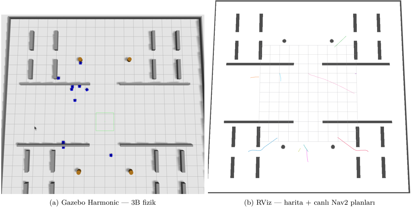
Fig. 7. En büyük (10-robot) dağıtımın AHE-MRTA altında bir dynamic_task_arrival örneğinde koşma anında alınmış canlı anlık görüntüsü. (a) Gazebo Harmonic 3B fizik: on TurtleBot3 Waffle Pi robotu (mavi) 20×20 m denetim arenasına—bölme duvarları, kare sütunlar ve silindir engeller (turuncu)—dağılmış, her biri atanmış bir denetim noktasına ilerliyor. (b) Eşzamanlı RViz görünümü (paylaşılan harita çerçevesinde): önceden oluşturulmuş işgal haritası, her robotun güncel Nav2 küresel planı (robot başına bir renk) ve ground-truth pozuyla bindirilmiş. Renk-kodlu planlar filonun her iki şeride yayıldığını gösterir—ekosistemin olay-başına, iş-koruyan dağıtımının görsel imzası.
