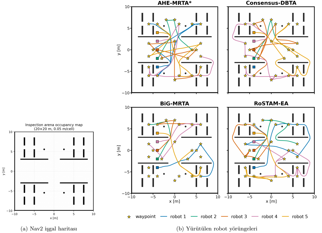
Fig. 6. Deney haritası ve örnek yörüngeler. (a) Statik Nav2 işgal haritası ( obstacle_map ) 20 \times 20 m, 0.05 m hücreli ve orijini [-10, -10] . İçinde ayırıcı duvarlar, kare sütunlar ve dört silindirik engel var. (b) Tek bir mixed_stress koşusundan (5 robot, 25 görev, tohum 1) AHE-MRTA, Consensus-DBTA, BiG-MRTA ve RoSTAM-EA yörüngeleri; sol üstten okuma sırasıyla. Bunlar, Tablo VII'daki 5r/25g mixed_stress hücrelerine giren dört koşunun ta kendisi. Kareler spawn konumları, altın yıldızlar örneklenmiş görev noktaları, renkli eğriler ise ground-truth pozlarından yeniden kurulmuş yollar. Zaman serisi her pozu robotun kendi odom çerçevesinde kaydettiği için her yörünge o robotun spawn noktası kadar ötelenmiştir. Eğrisiz bir kare, spawn noktasından hiç ayrılmamış bir robottur; burada Consensus-DBTA'nın robot 1'i böyledir. Bu tek koşuluk figür niteliksel; toplu bir yöntem sıralaması ortaya koymaz.
