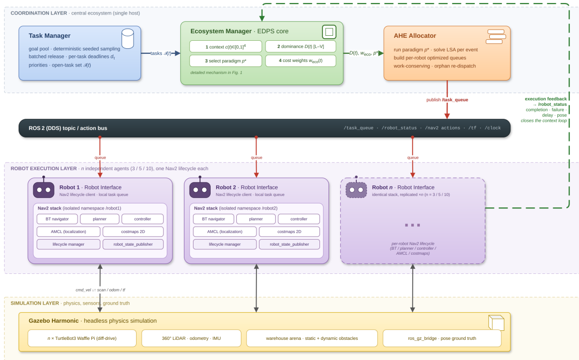
Fig. 2. Sistem mimarisi. Ekosistem yöneticisi hormon durumunu günceller, etkin paradigmayı seçer ve ROS2 konuları ile her robot için bir görev kuyruğu yayımlar. Her robot kendi Nav2 yaşam döngüsünü çalıştırır ve tamamlama, arıza ve gecikme geri bildirimini yöneticiye gönderir.
