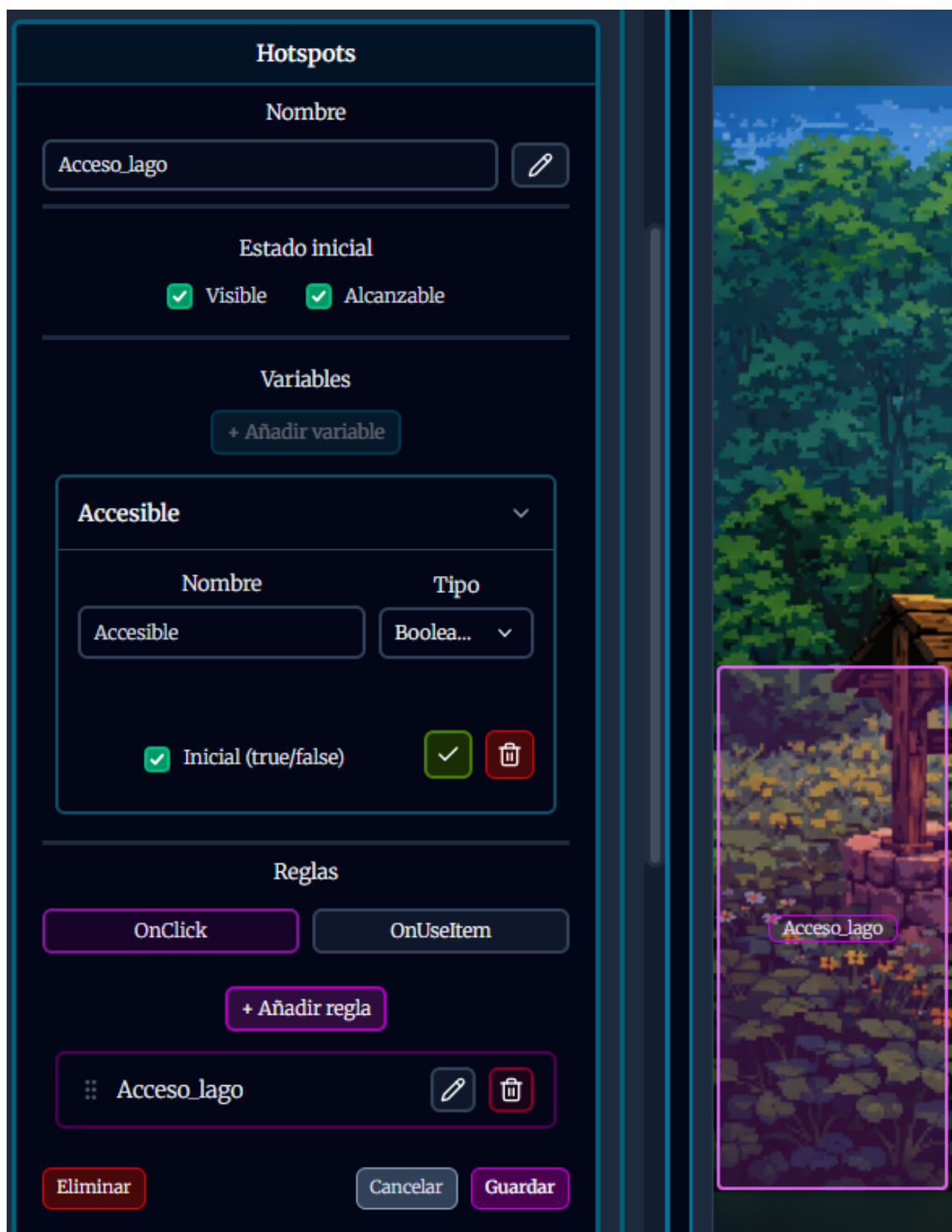
Figura 1.7: Configuración de un elemento interactivo
