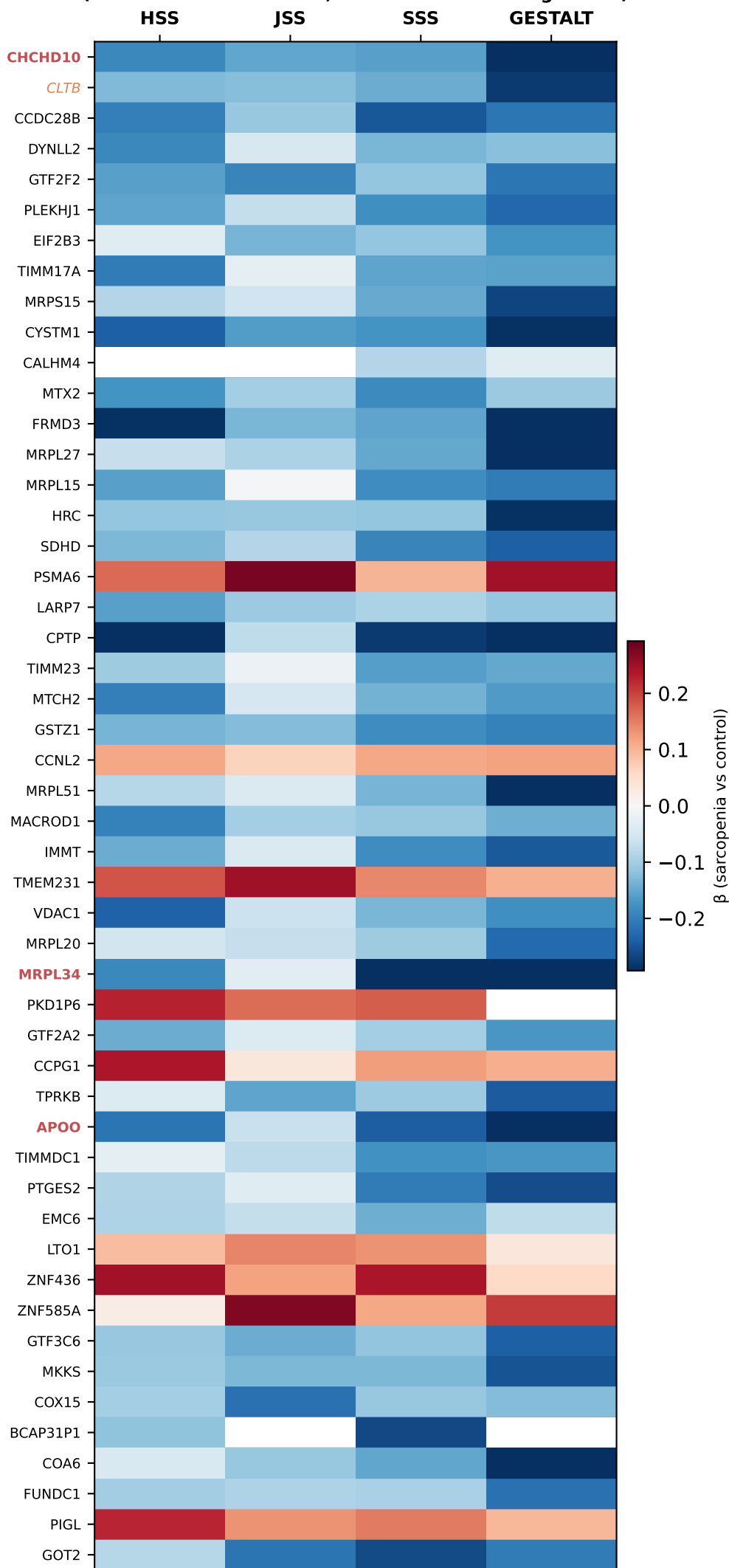
Figure 4. Top 50 candidate genes (mitochondrial: red bold; CLTB non-mito: orange italic)
