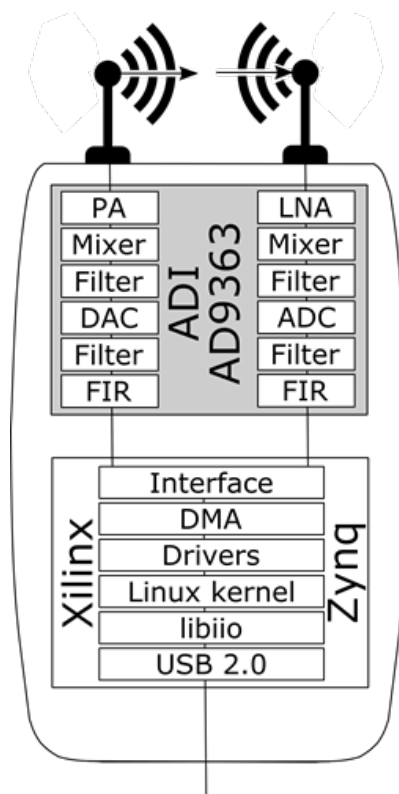
Рисунок 1 — Архитектура ADALM-Pluto (схема)
