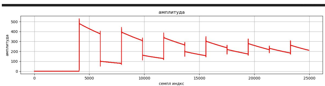
Рисунок 12 — График амплитуды принятого сигнала (RX). Наблюдается ослабление и искажение сигнала по сравнению с переданным, что объясняется характеристиками радиоканала и фильтрации в устройстве.
