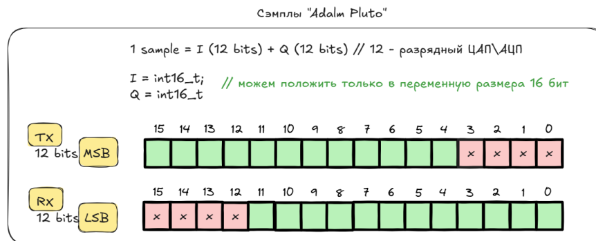
Рисунок 14 — Структура сэмпла ADALM Pluto. Каждый сэмпл состоит из 12-битных значений I и Q. При работе с 16-битными переменными ( int16_t ) для TX используется старшие 12 бит (MSB), а для RX — младшие 12 бит (LSB).
