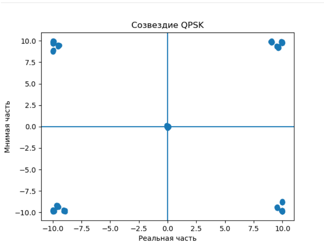
Рисунок 26 — Созвездие принятого сигнала после синхронизации. Точки сконцентрированы в четырёх кластерах, что соответствует символам QPSK.
