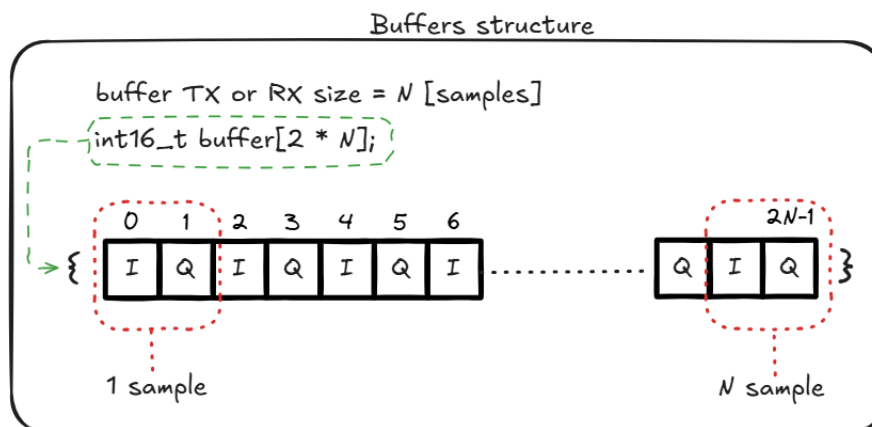
Рисунок 8 — Структура буфера для TX/RX потоков. Массив типа int16_t длиной 2 \cdot N хранит N комплексных сэмплов, где каждый сэмпл представлен парой значений I и Q.
