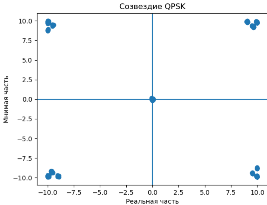
Рисунок 26 — Созвездие принятого сигнала после синхронизации. Точки сконцентрированы в четырёх кластерах, что соответствует символам QPSK.
