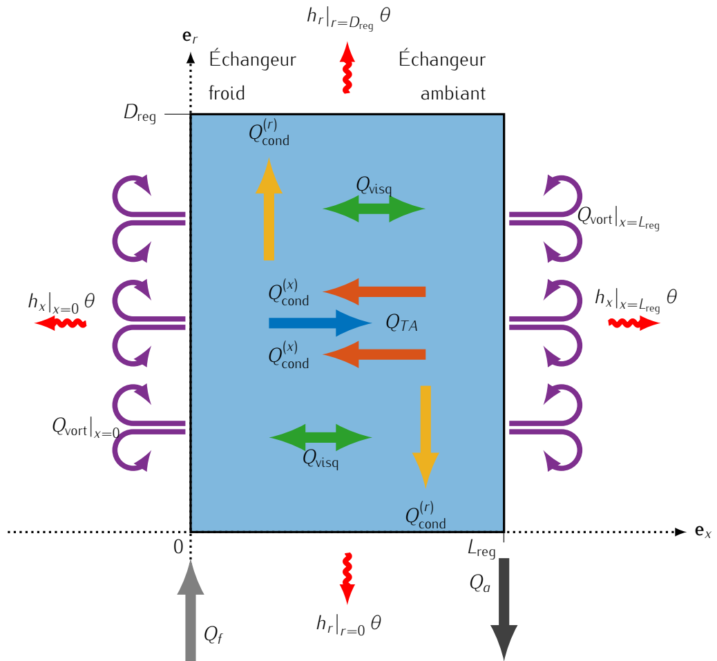
FIGURE 1 – Représentation schématique des flux thermiques considérés dans le modèle transitoire du régénérateur.
