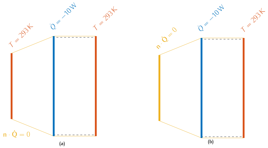
FIGURE 1 – Conditions aux frontières thermiques. Le côté ambiant du régénérateur est à température fixée, le côté froid est modélisé par un puit de chaleur, et la paroi de la source acoustique principale est modélisée par deux conditions asymptotiques. (a) température ambiante, et (b) adiabatique.
