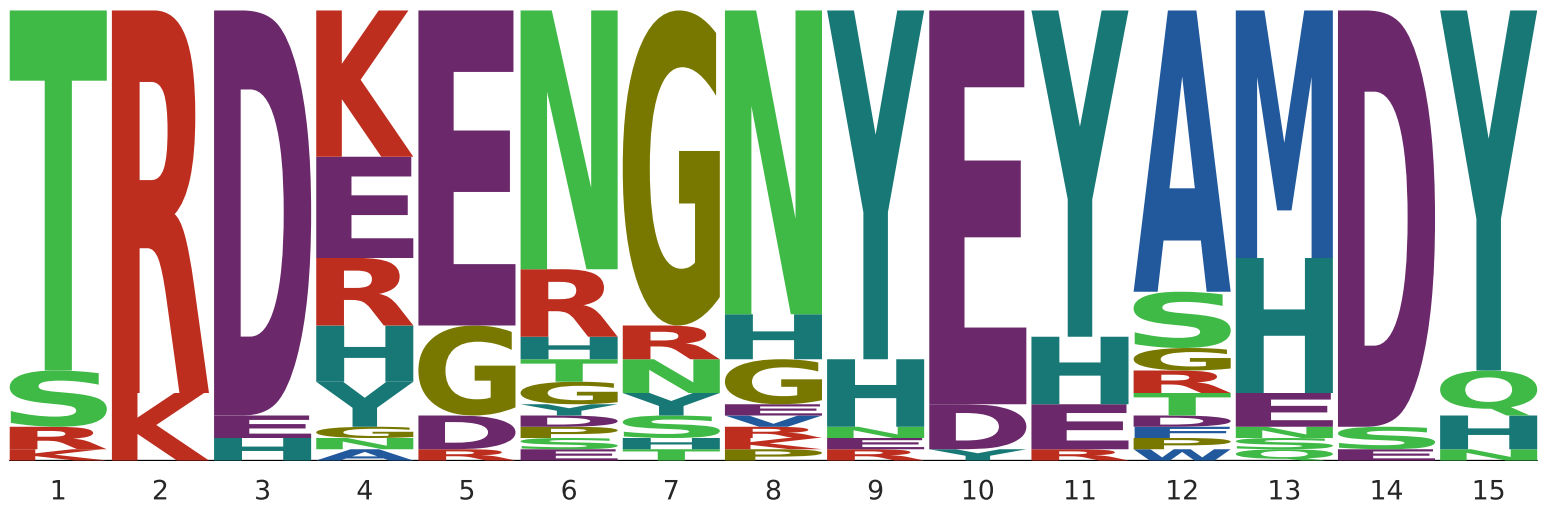
2JEL
