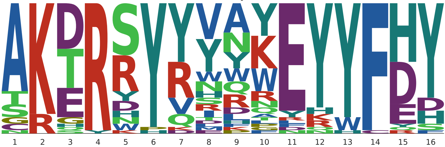
1NSN
