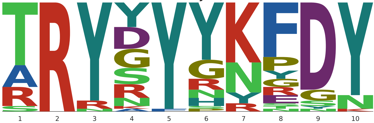
3VRL
