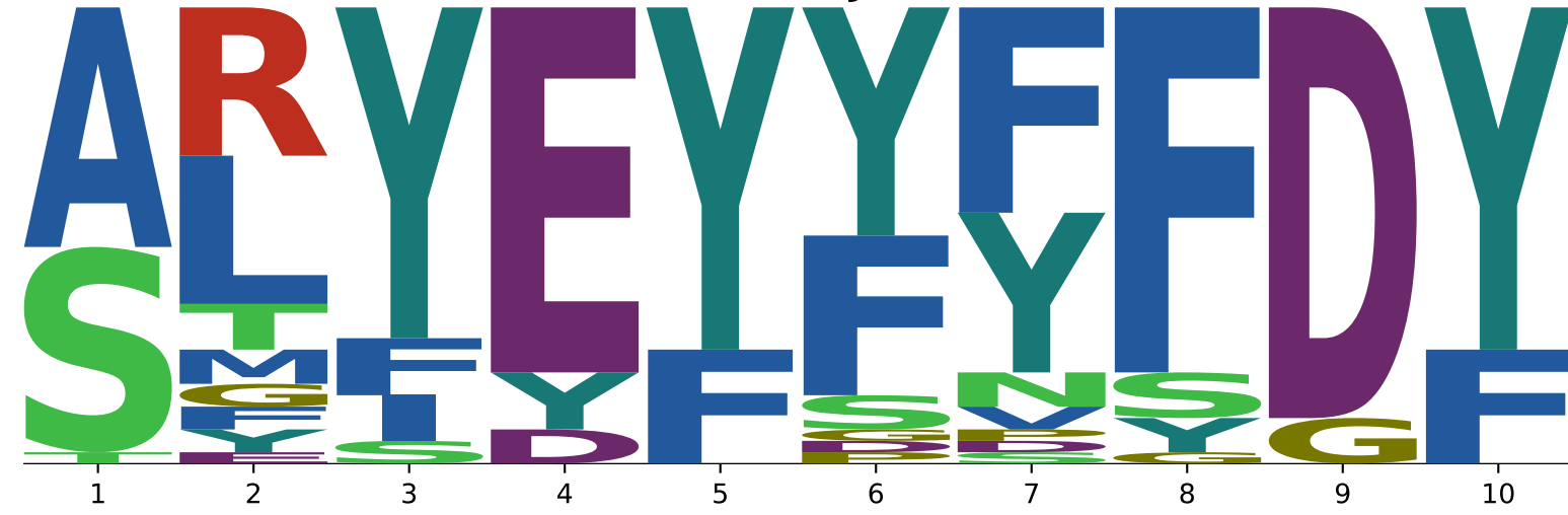
3VRL
