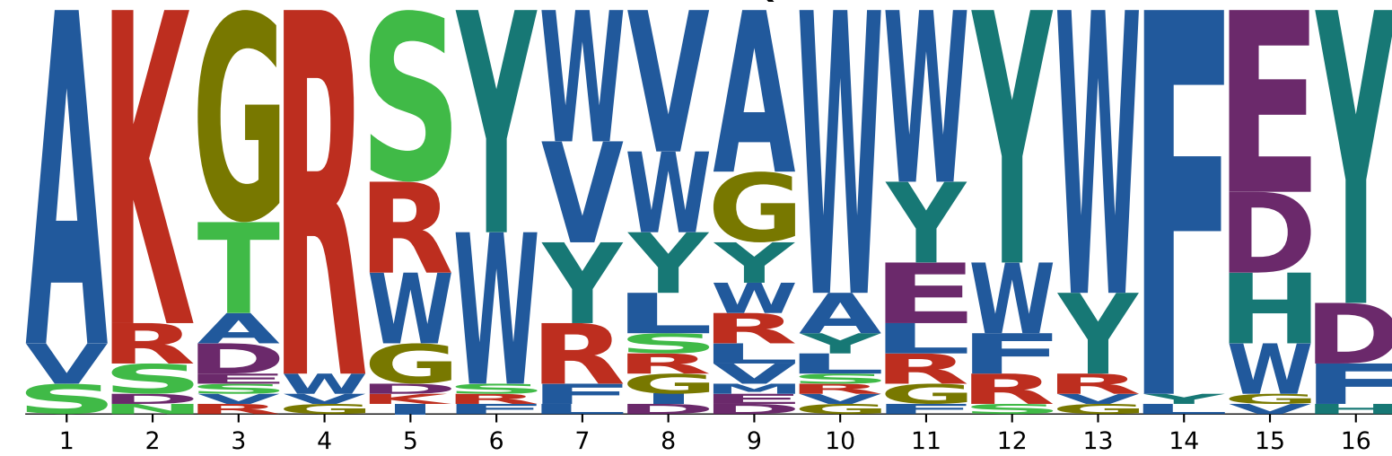
1NSN
