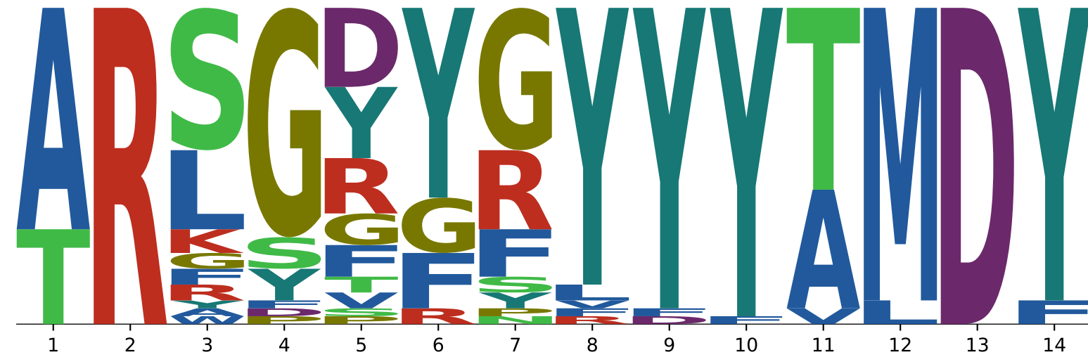
1WEJ
