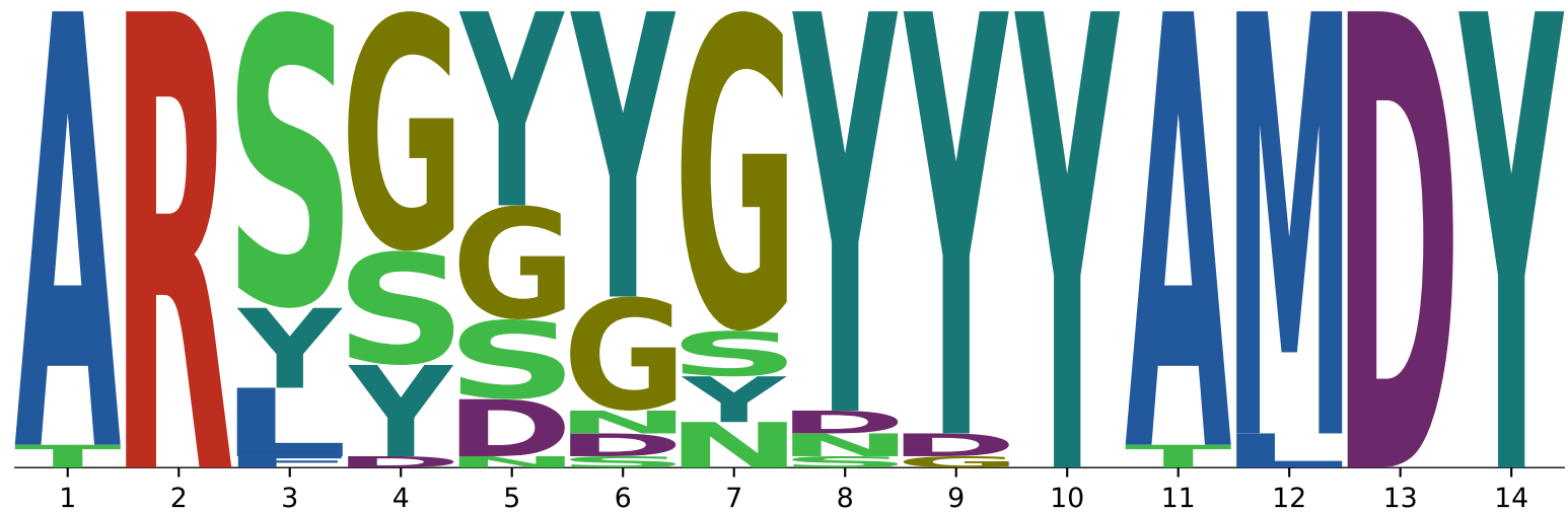
1WEJ
