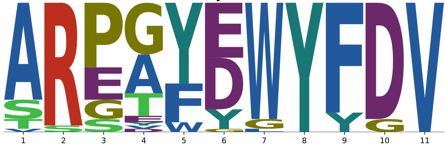
2JEL
