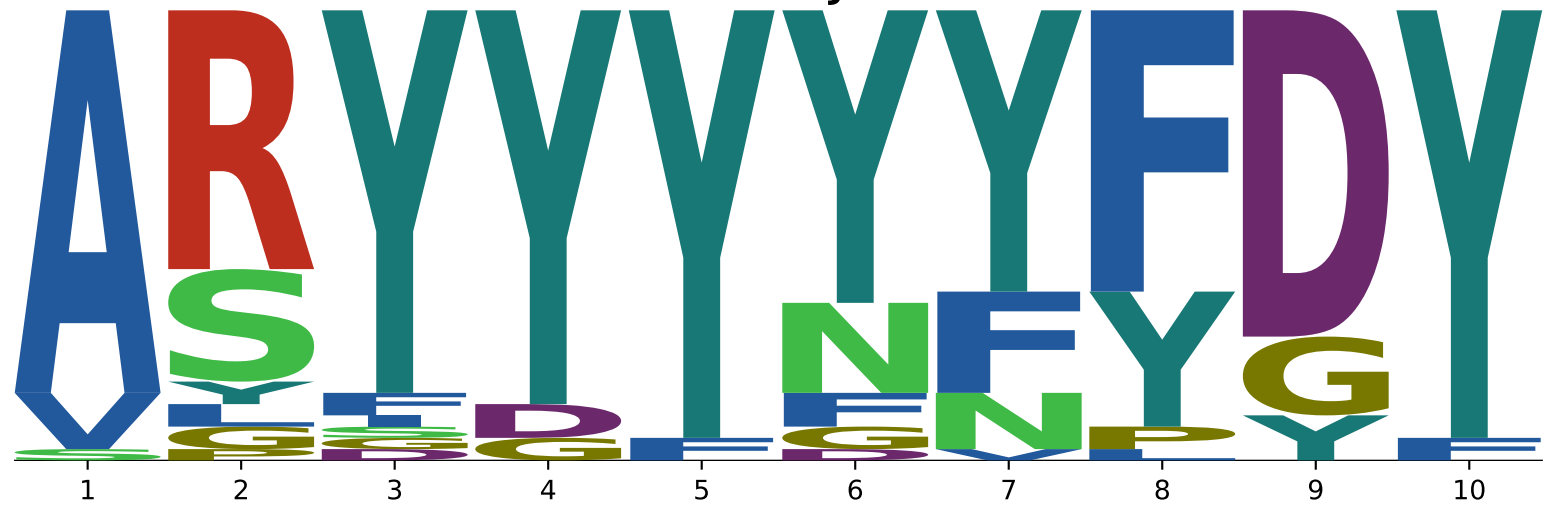
3VRL
