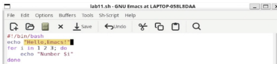
Рисунок 5: Пример удаления строки с помощью C-k
