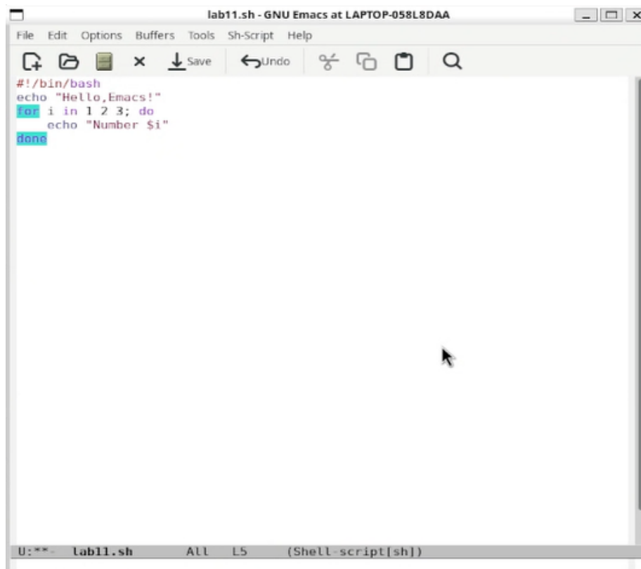
Рисунок 3: Создание нового файла
