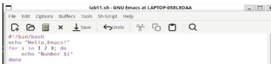
Рисунок 4: Буфер с введённым текстом
