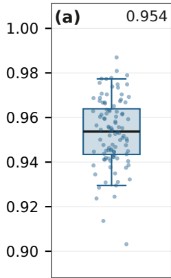
AUROC
