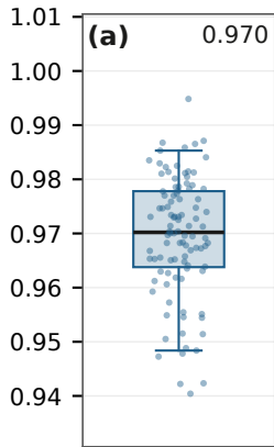
AUROC
