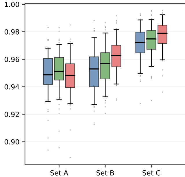
AUROC
