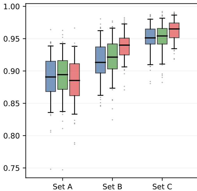
AP (PR-AUC)
