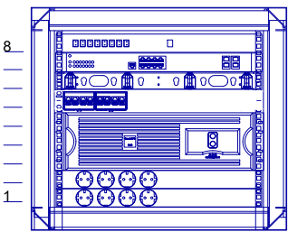
Коммуникационный шкаф 8U(XB-01)
