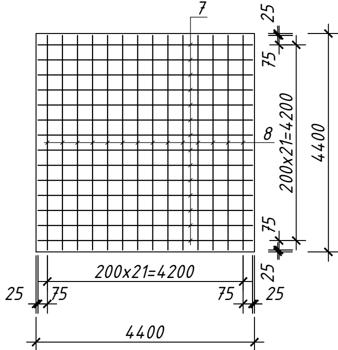
Арматурная сетка С-4 М1:50
