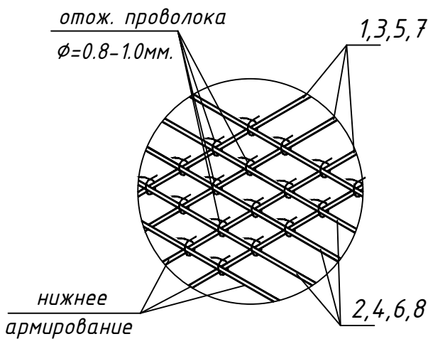
Деталь установки арм.сетки
