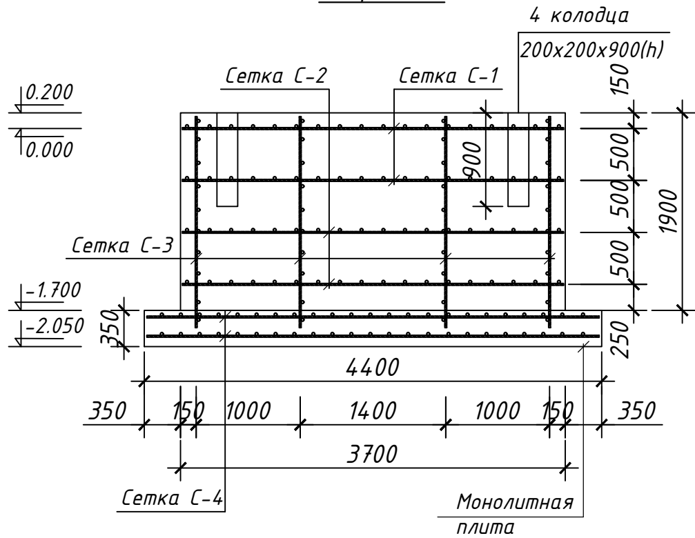
Разрез 1-1
