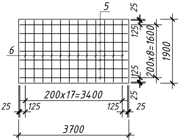
Арматурная сетка С-3 М1:50
