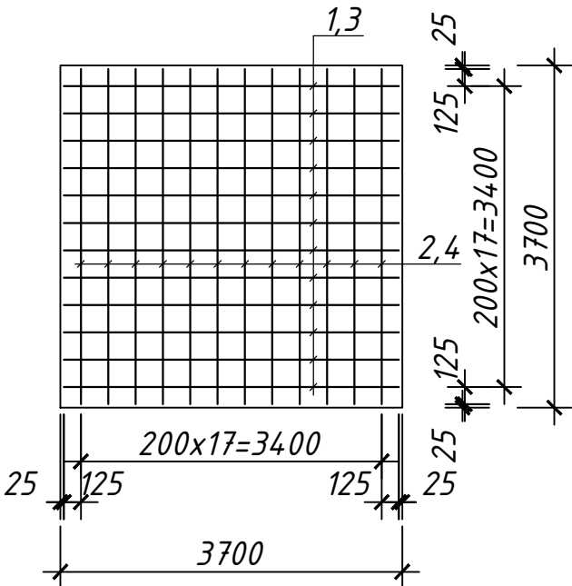
Арматурная сетка С-1 (С-2) М1:50
