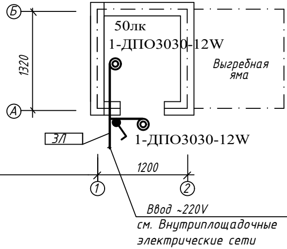
План сети электроосвещения. 1:100
