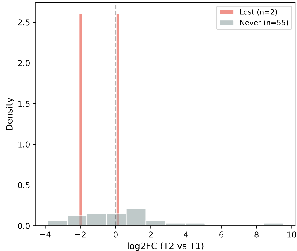
A) T1→T2 (MTase drops) p=4.52e-01
