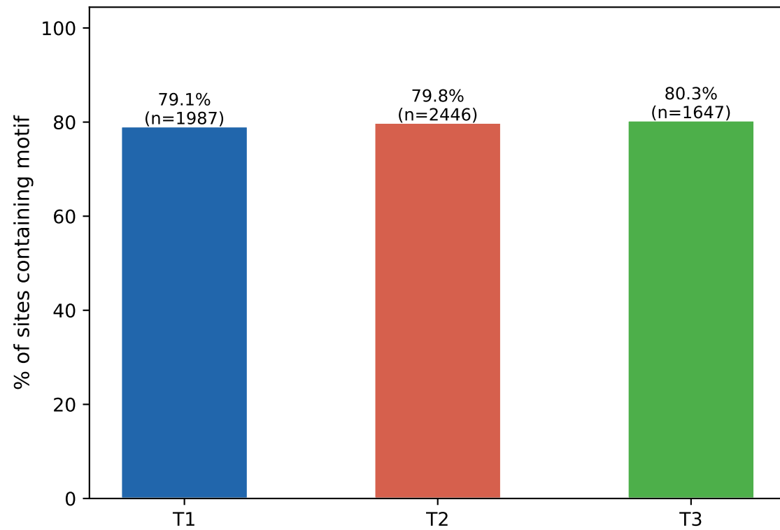
6mA — TCGA
