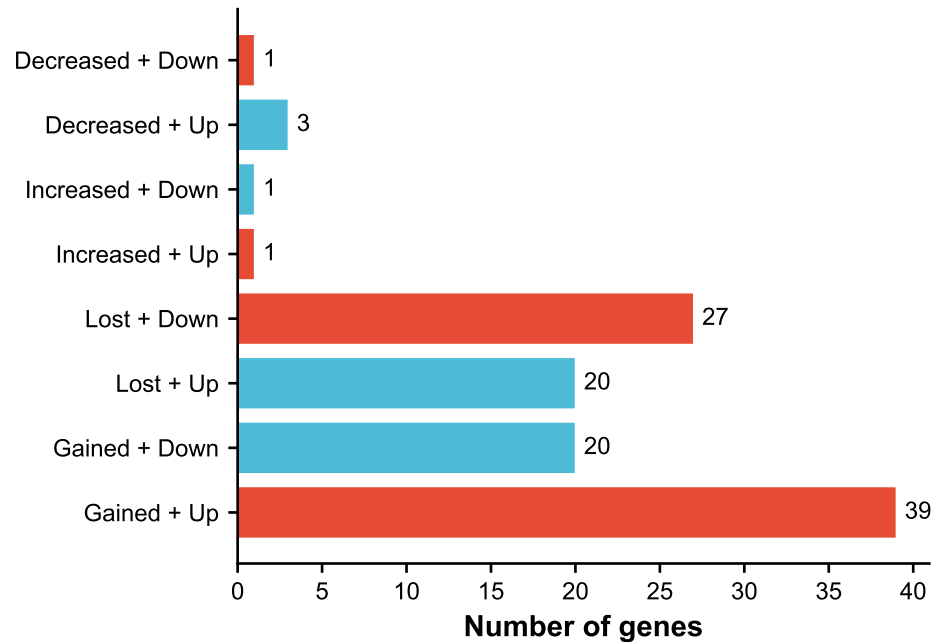
6mA
