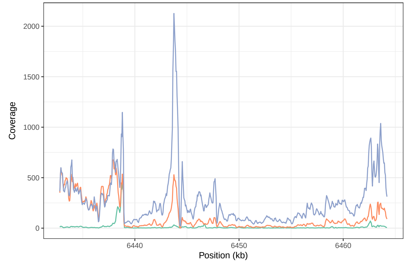
cpk (Coelimycin P1)
