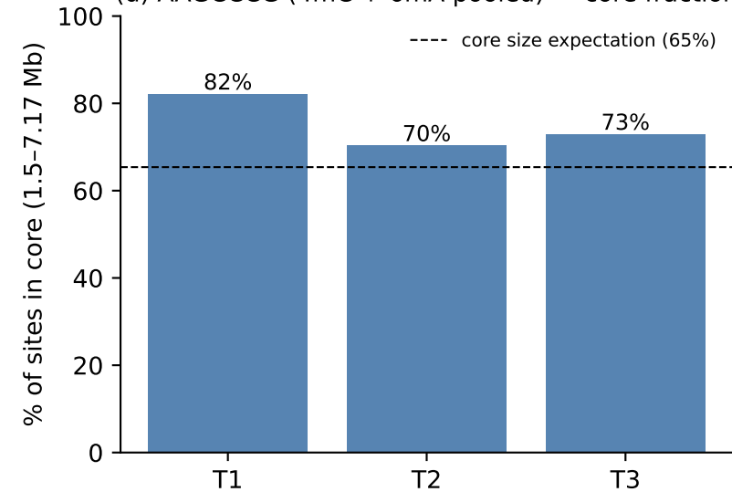
(d) AAGCCCG (4mC + 6mA pooled) — core fraction
