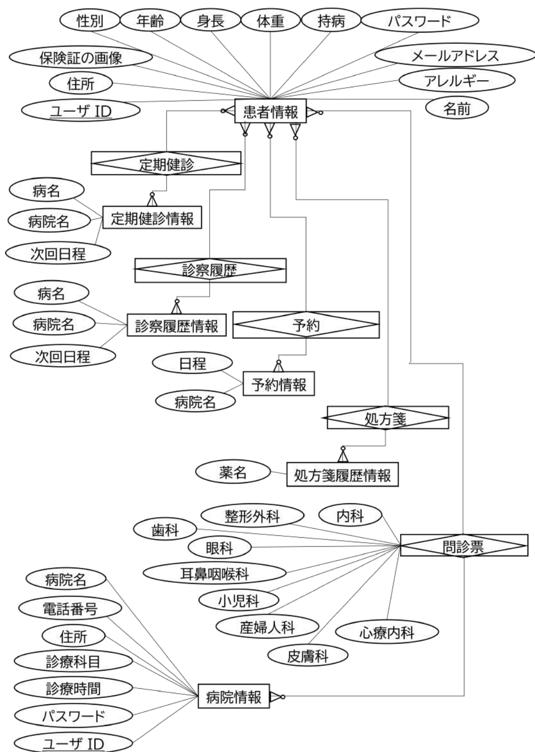
図 44 ER 図
