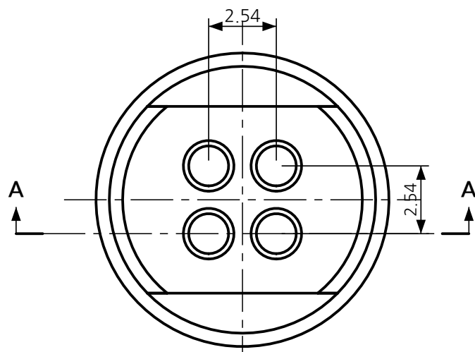
윗면도 (센서 소켓 쪽)
