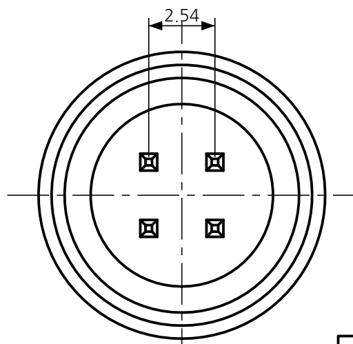
아랫면도 (PCB 핀 쪽)
