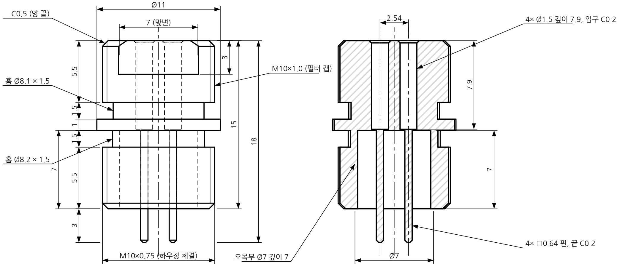
정면도
