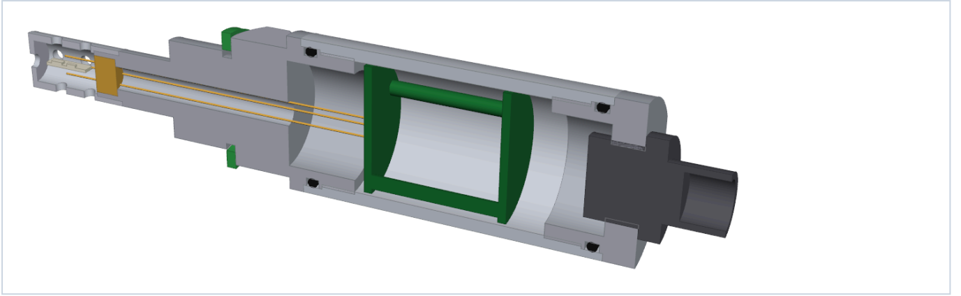
Rev B 3D 단면: 바디-하우징-엔드캡 M28×1 나사 + O링 결합, 커넥터 전면 장착
