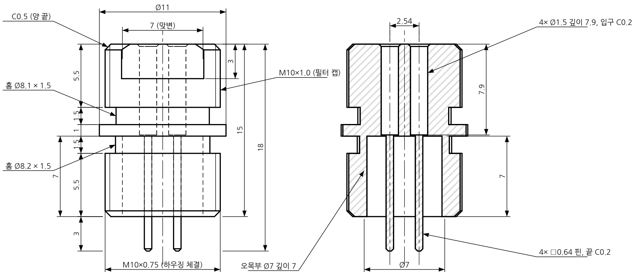
정면도
