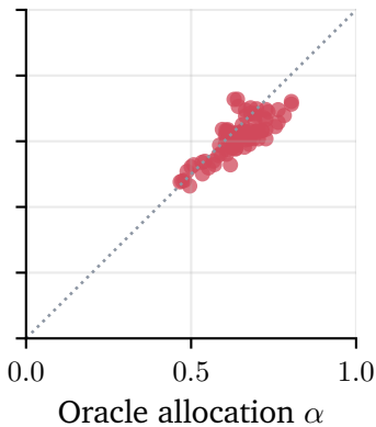
MLP
