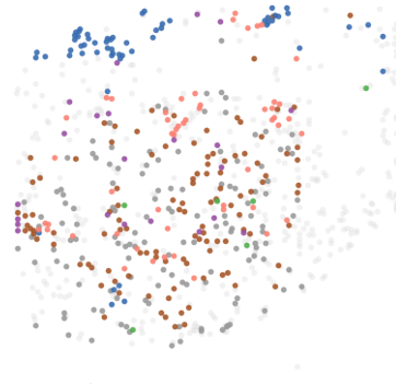
MIBI · human glioma (1 FOV)
