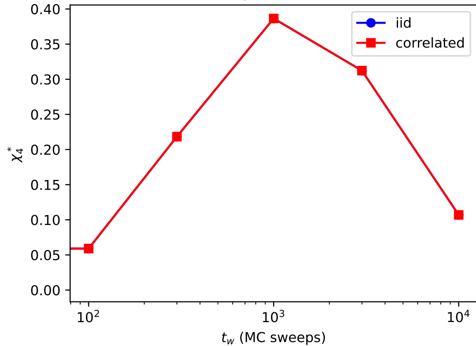
epsilon=0
