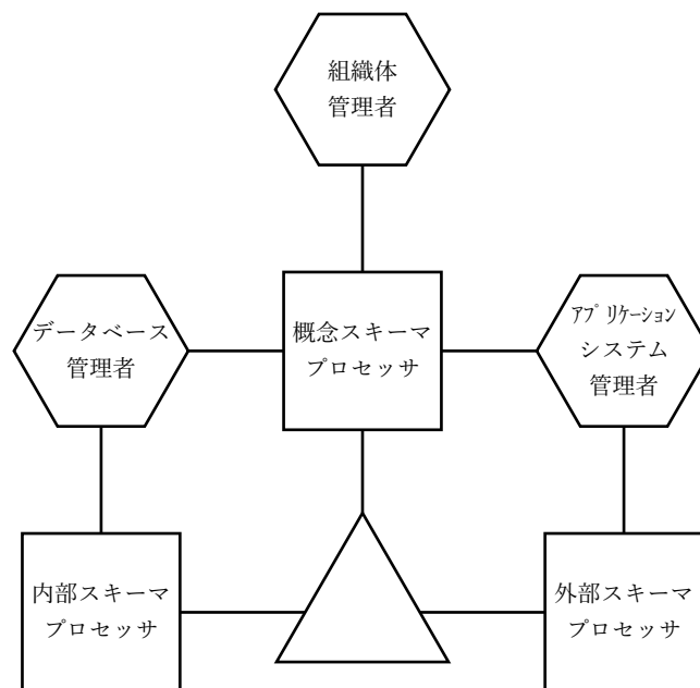
図 7.1: ANSI/X3/SPARC の DBMS3 層スキーマ構造の一部
