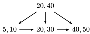
図 7.3: B + 木の例
