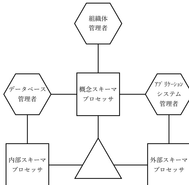
図 7.1: ANSI/X3/SPARC の DBMS3 層スキーマ構造の一部
