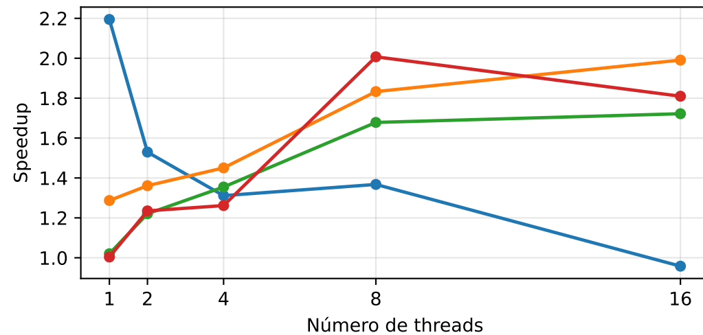
Pthreads EM
