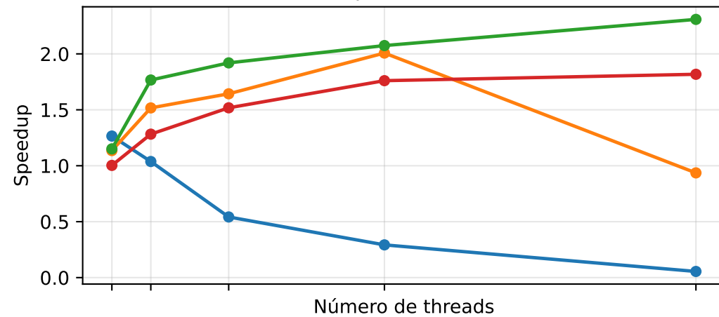
Pthreads EM
