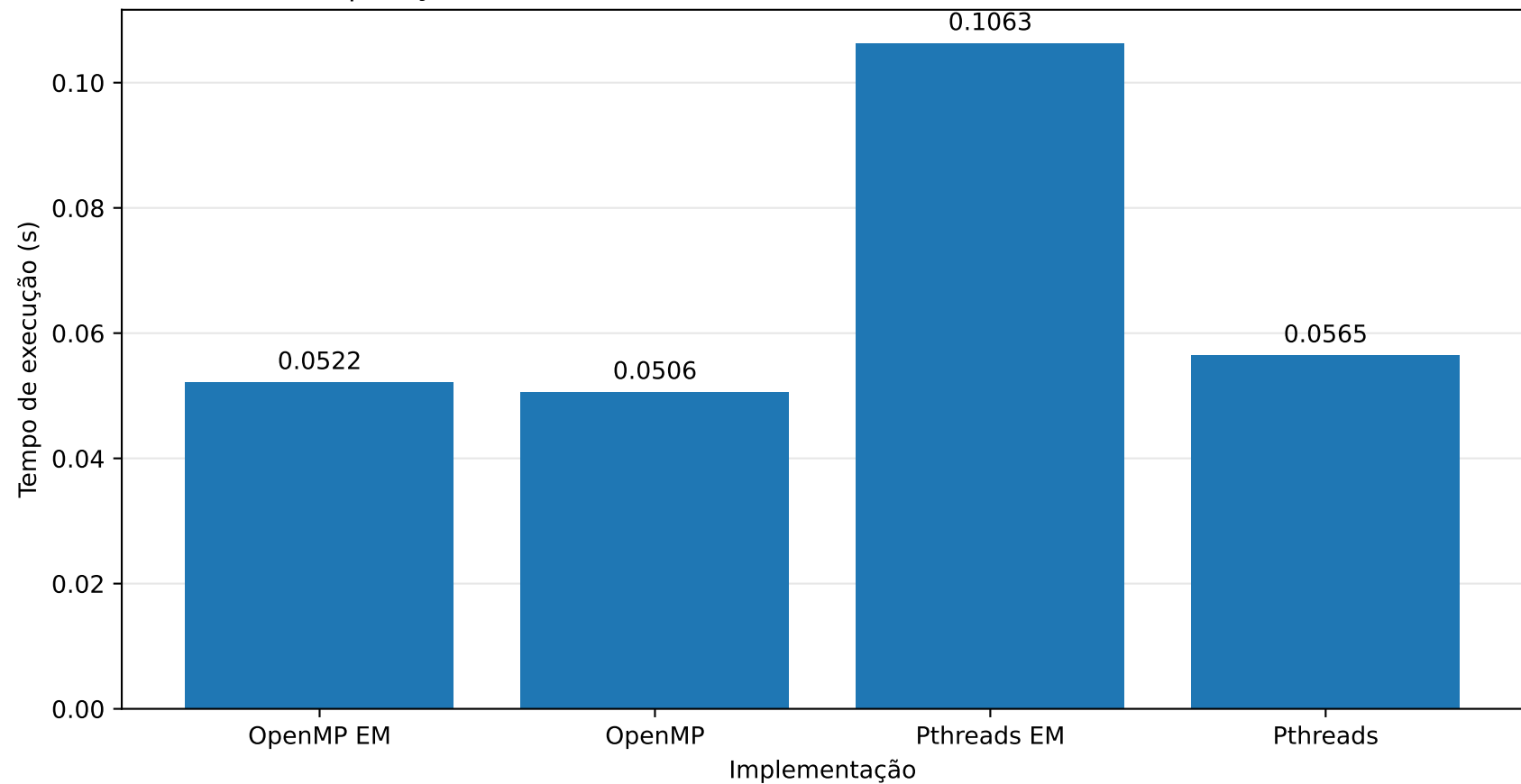
Comparação com e sem exclusão mútua — 5.000 vértices, 40%, 8 threads
