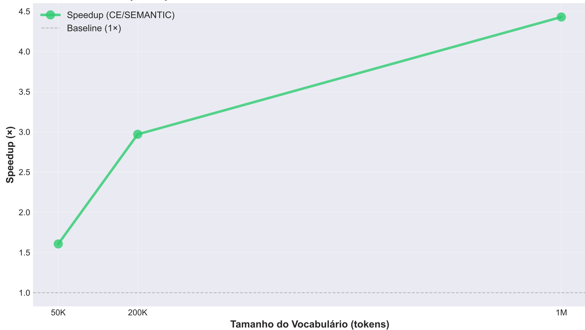
Speedup do OktoSemantic vs Tamanho do Vocabulário - RTX A6000
