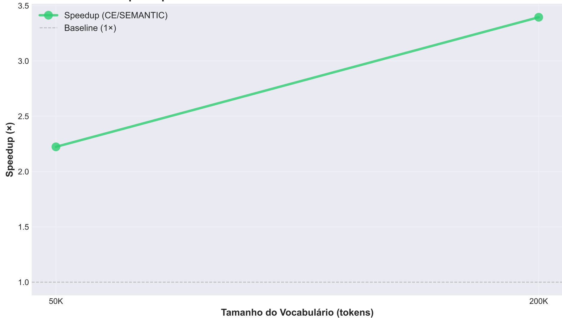
Speedup do OktoSemantic vs Tamanho do Vocabulário - RTX 4070
