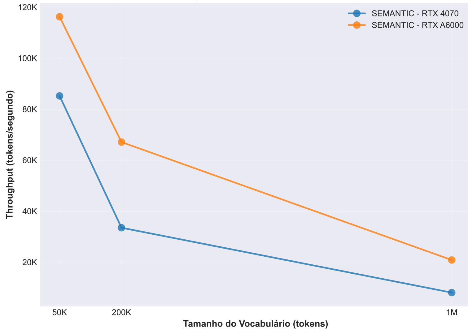
Throughput: Comparação entre GPUs
