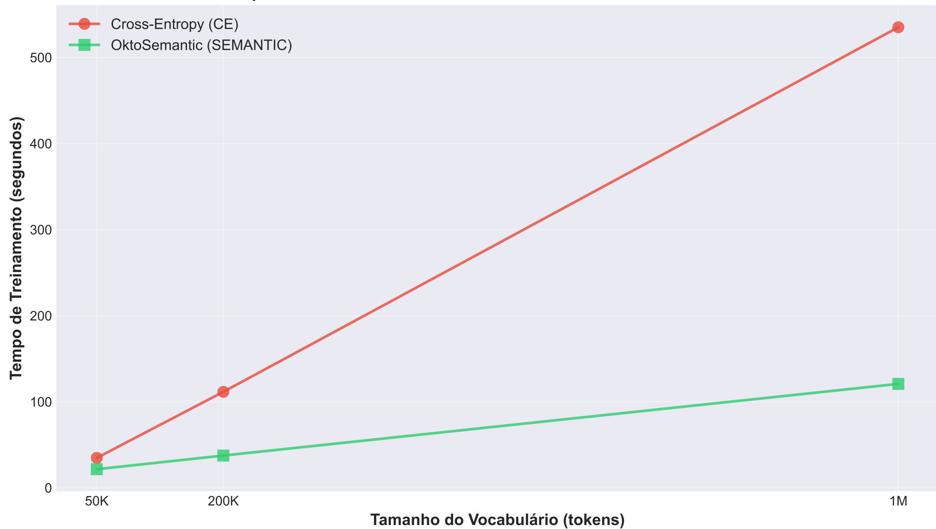
Tempo de Treinamento vs Tamanho do Vocabulário - RTX A6000
