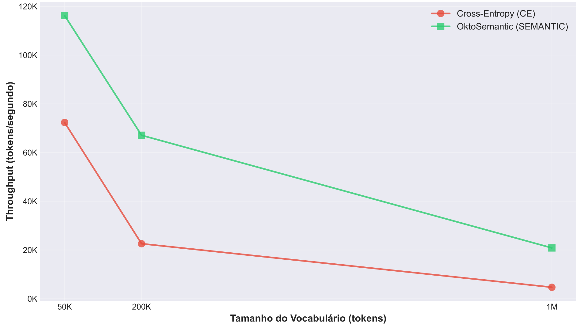
Throughput vs Tamanho do Vocabulário - RTX A6000
