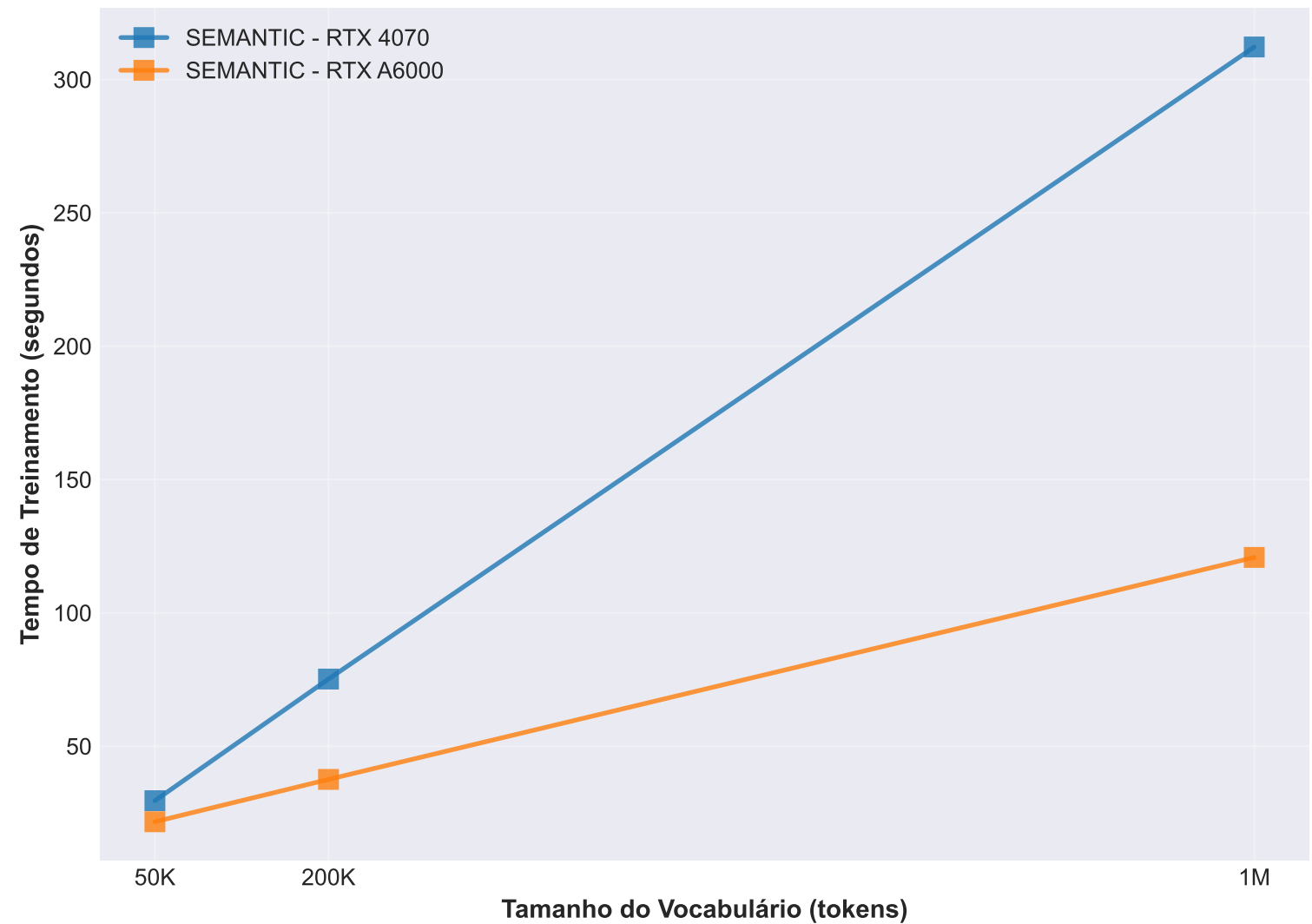
Tempo de Treinamento: Comparação entre GPUs
