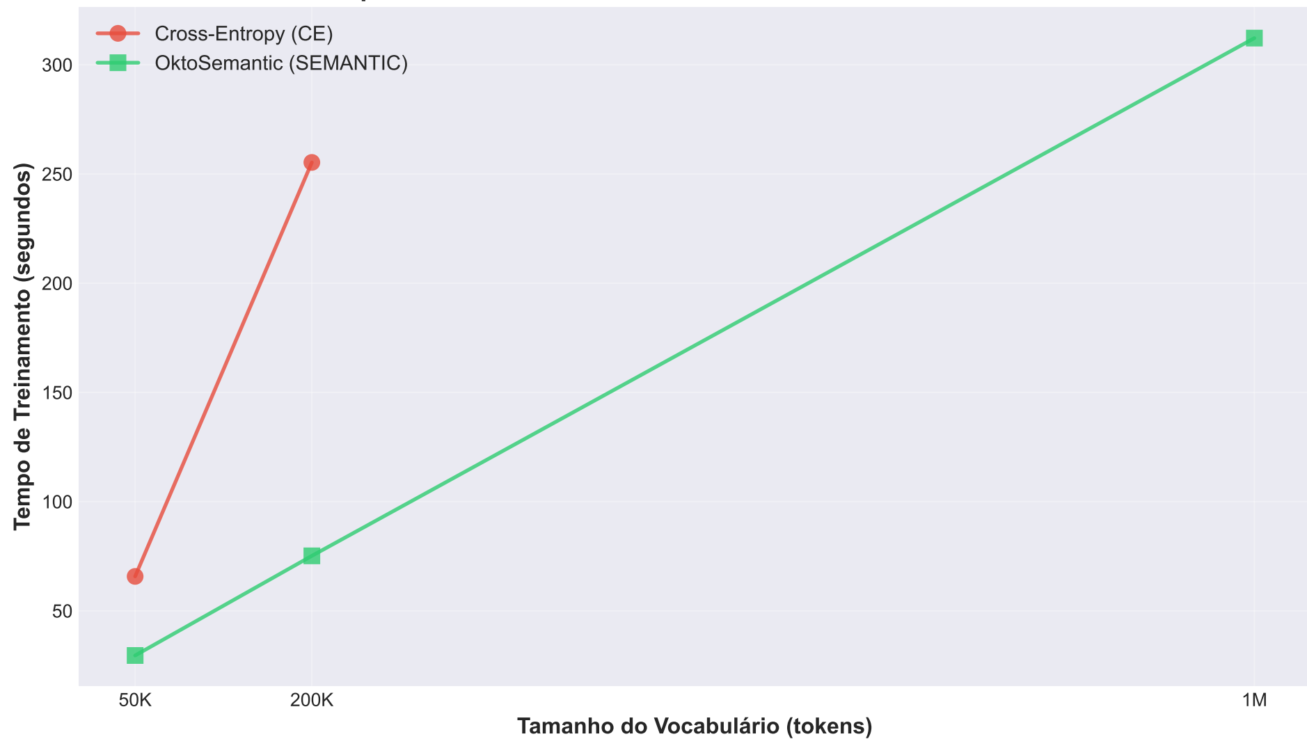
Tempo de Treinamento vs Tamanho do Vocabulário - RTX 4070
