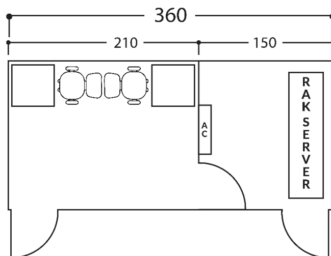
DENAH RUANG IT BARU (SKENARIO 2)
