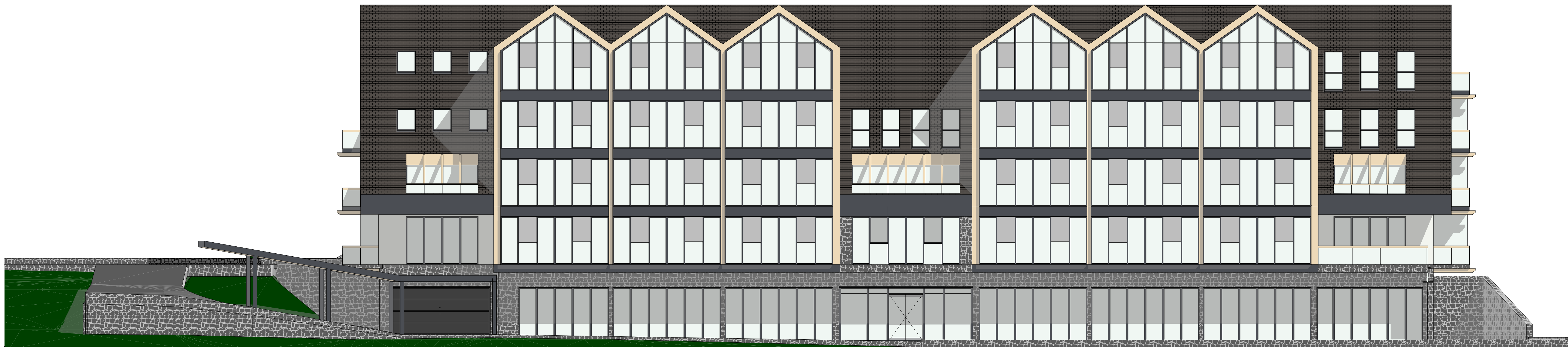
ELEWACJA POŁUDNIOWA
