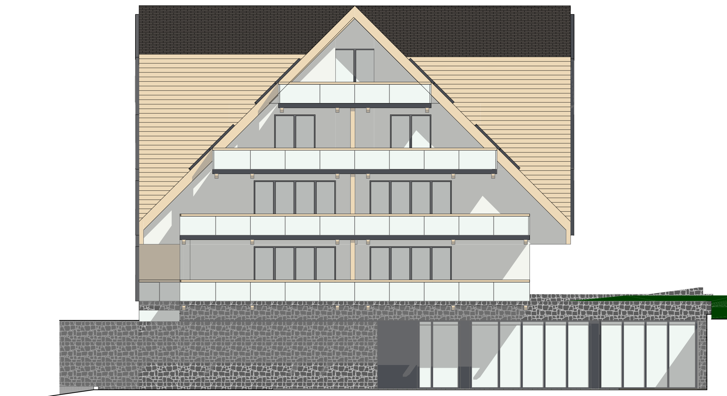
ELEWACJA WSCHODNIA
