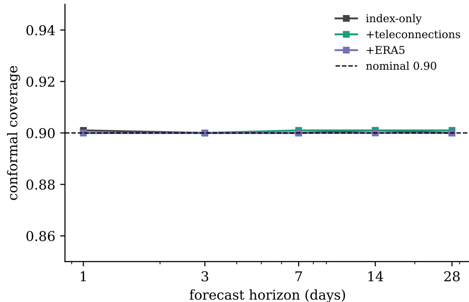
(d) Paris: calibration holds at all horizons
