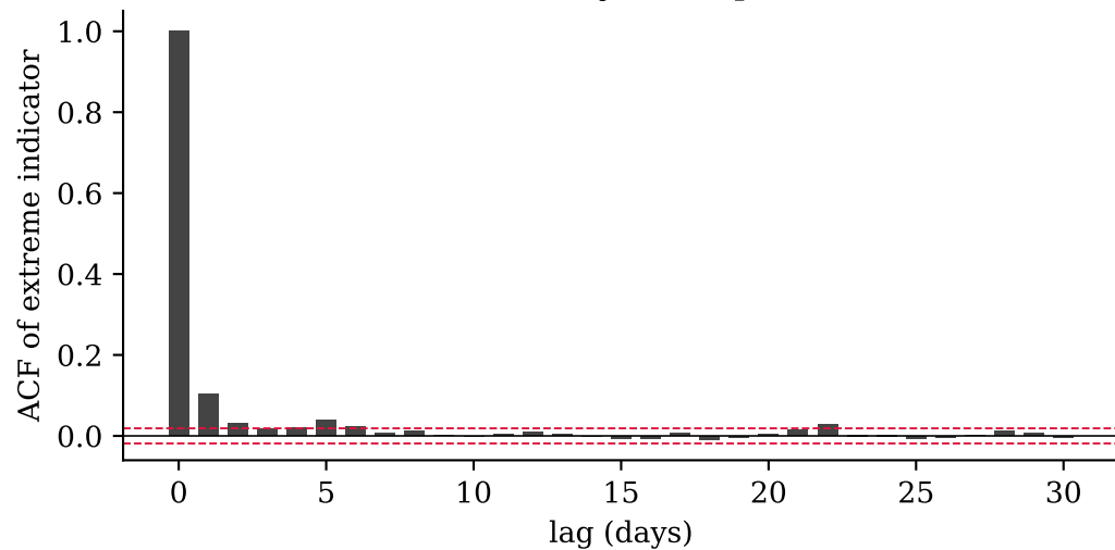
(d) Short memory: little persistence
