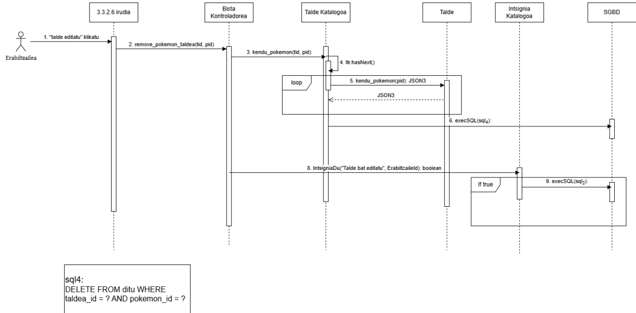
6.4.2.3 Irudia: Taldea editatzearen sekuentzia diagrama
