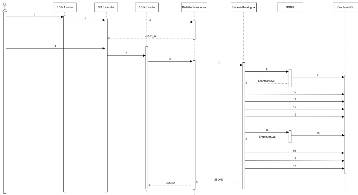
6.4.5.2 Irudia: ChatBot barneko "PokeMota" funtzionalitatearen Sekuentzia Diagrama
