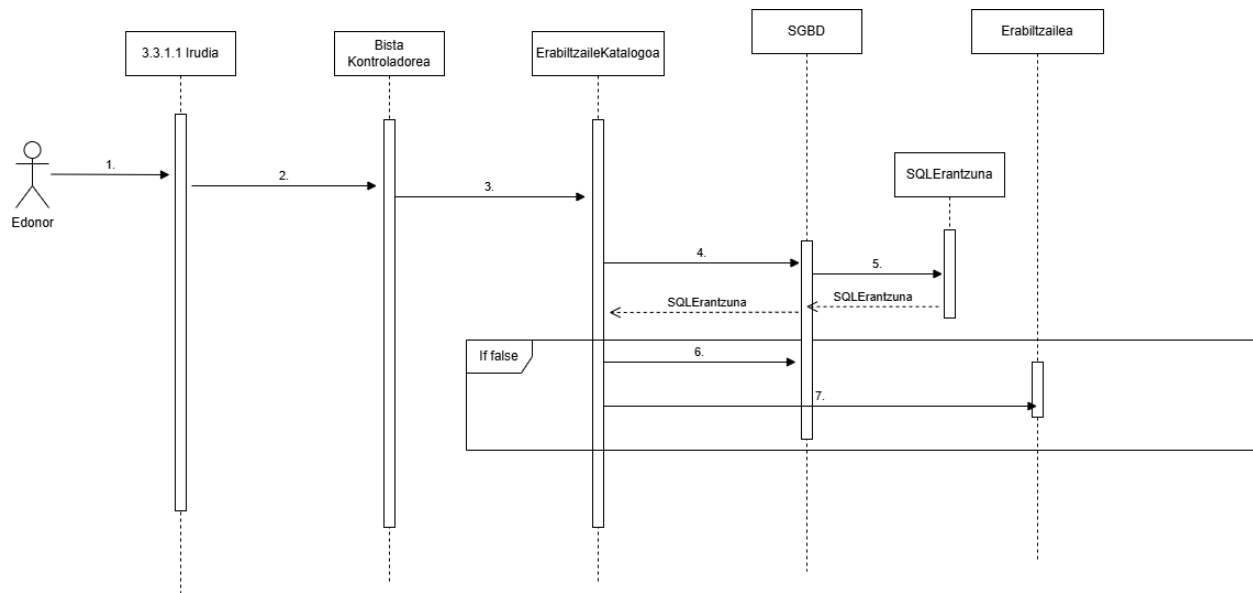
6.4.1.1 Irudia: Erabiltzailea erregistartzearen sekuentzia diagrama
