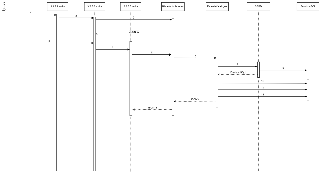
6.4.5.3 Irudia: ChatBot barneko "PokeEbo" funtzionalitatearen Sekuentzia Diagrama
