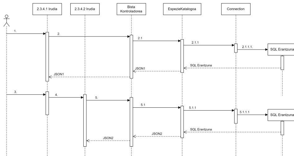
6.4.4 Irudia: Pokemonak zerrendatzea eta bilatzearen sekuentzia diagrama
