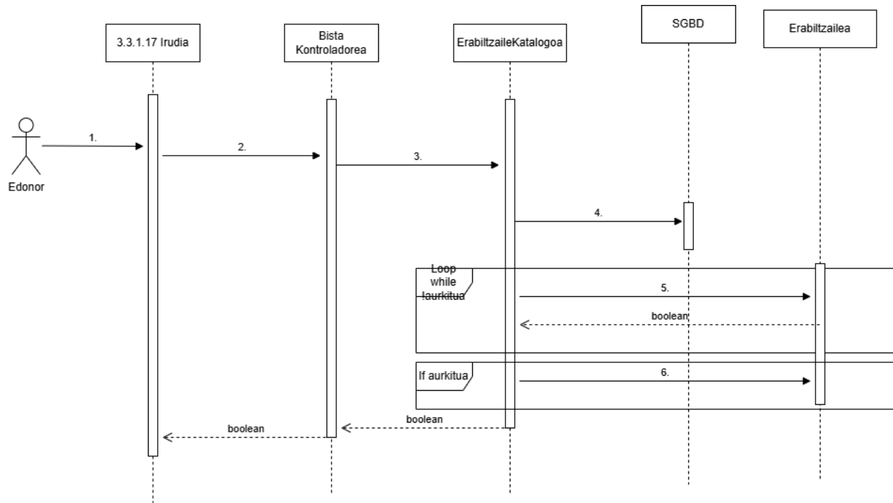
6.4.2.4 Irudia: Administratzaile bihurtzearen sekuentzia diagrama
