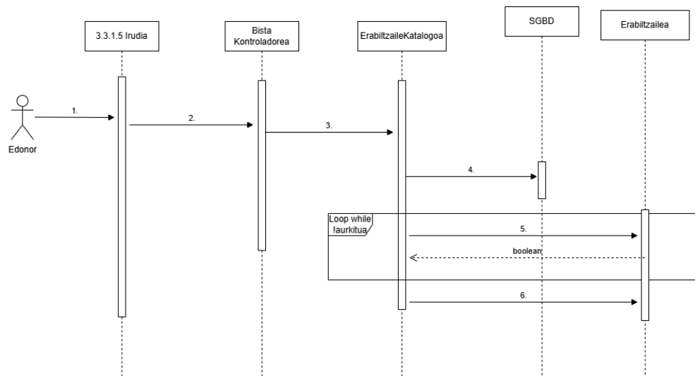
6.4.2.3 Irudia: Datuak eguneratzearen sekuentzia diagrama
