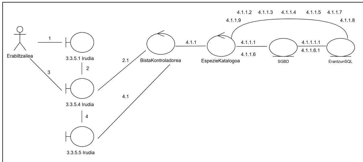
6.3.5.2.1 irudia: ChatBot menuan 'PokeMota' sakatzearen komunikazio diagrama
