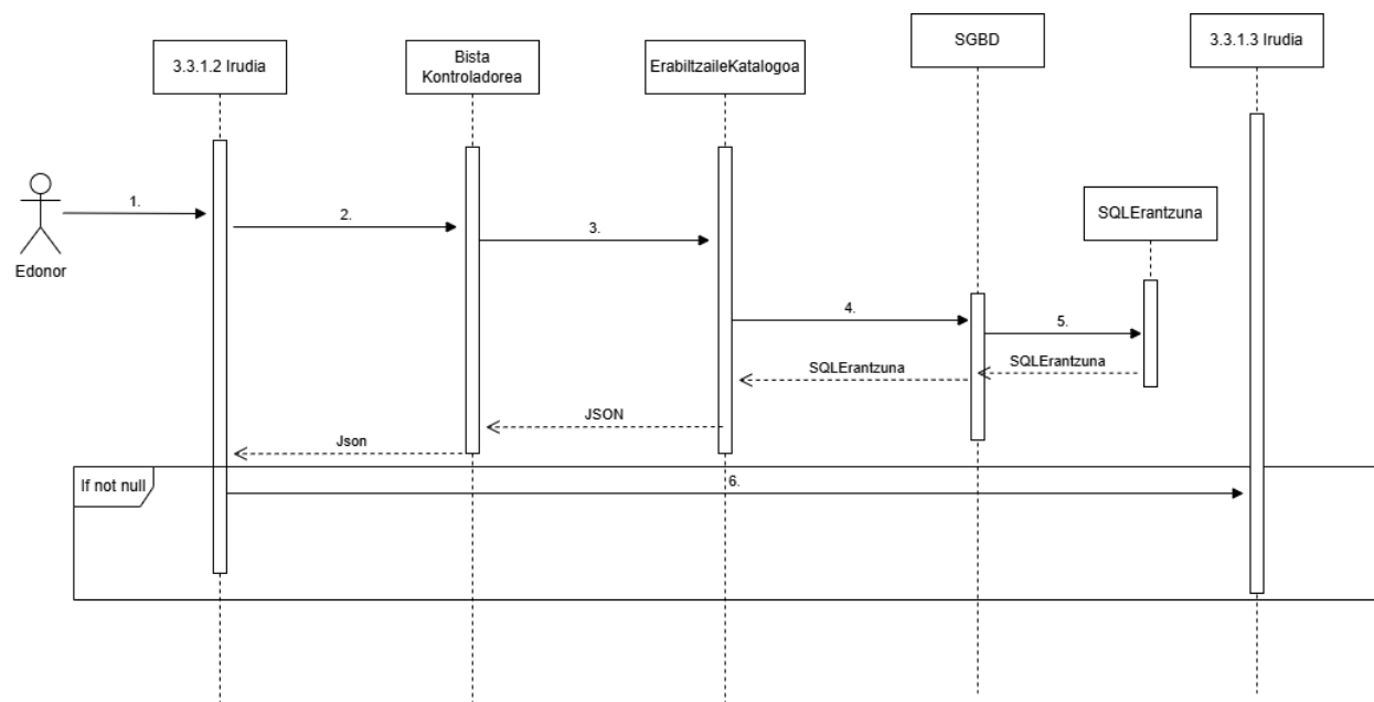
6.4.2.2 Irudia: Saioa hastearren sekuentzia diagrama
