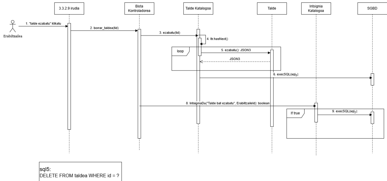
6.4.2.4 Irudia: Taldea ezabatzearen sekuentzia diagrama
