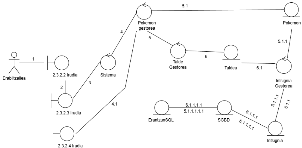
6.3.2.1.irudia: Taldea sortzeko komunikazio diagrama
