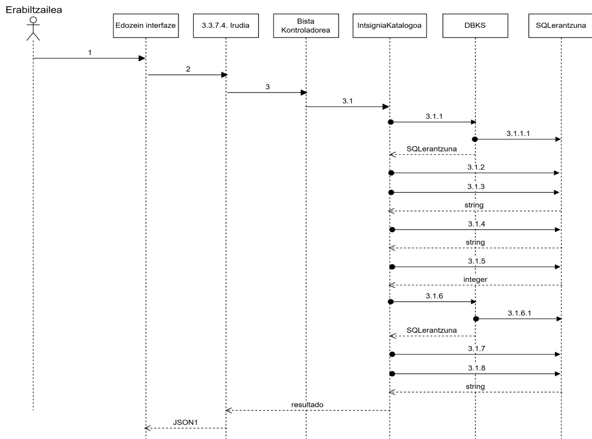
6.4.7.1 Irudia: Intsignien funtzionalitatearen barne logikaren Sekuentzia Diagrama
