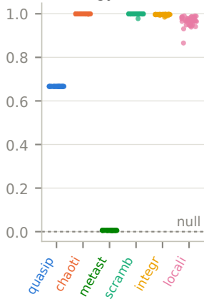
\Xi (energy coherence)
