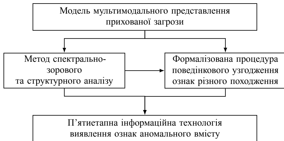
Рисунок 2.5 – Взаємозв'язок моделі, методу, формалізованої процедури та інформаційної технології
