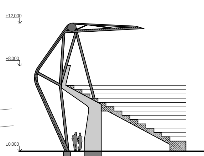
Розріз 1-1
