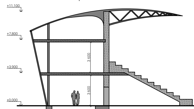
Розріз 2-2
