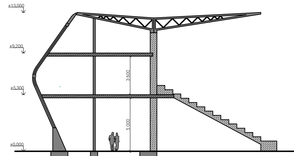
Розріз 2-2
