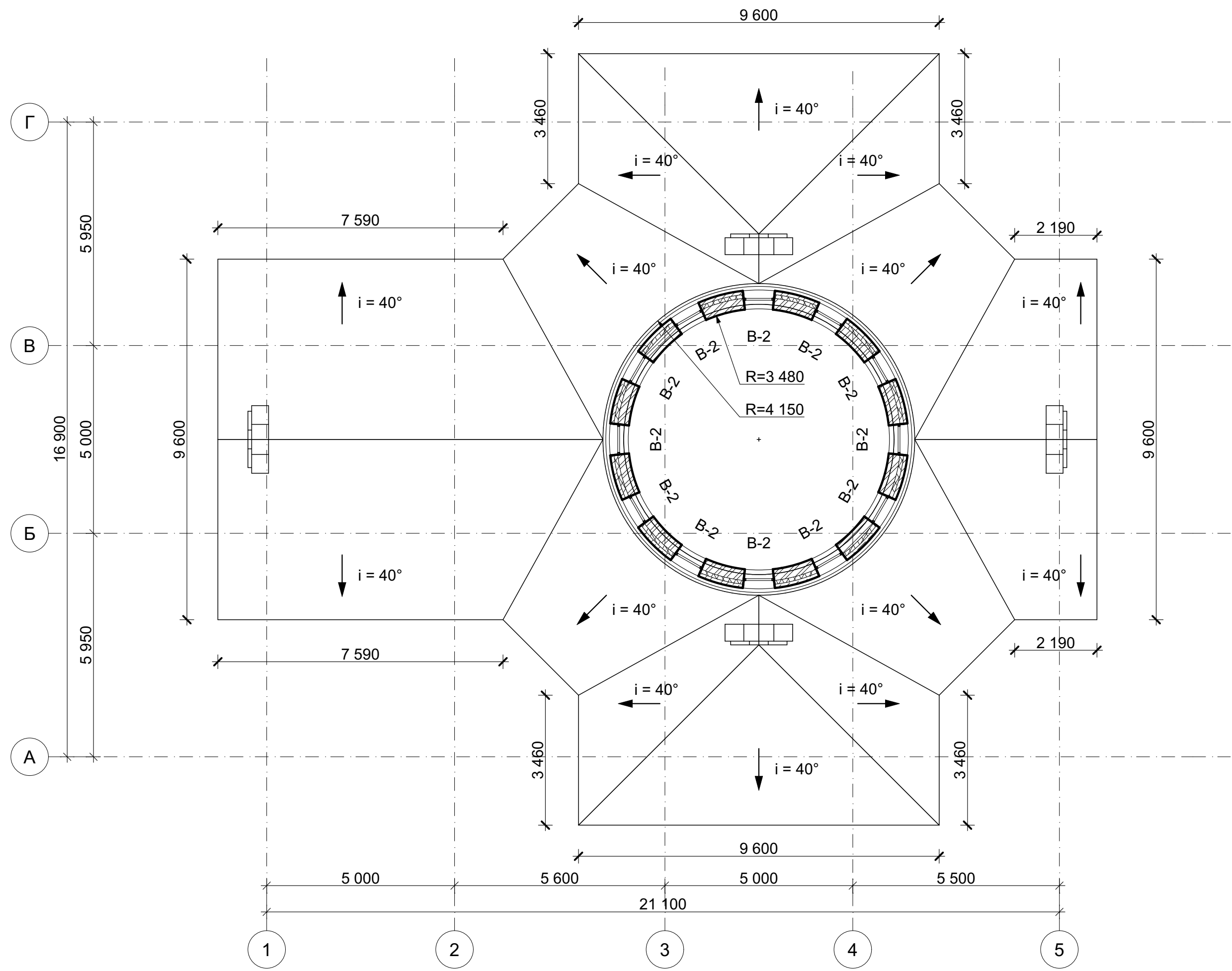
План даху М 1:100
