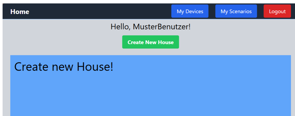
Abbildung 5: Leere Hauptseite
