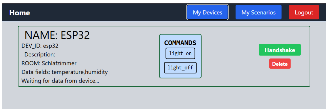
Abbildung 10: My Devices
