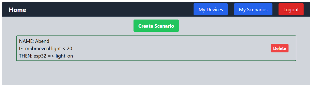
Abbildung 12: My Scenarios
