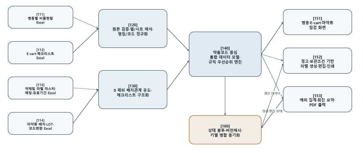
도 1. 전체 업무 앱의 데이터 처리 블록도
